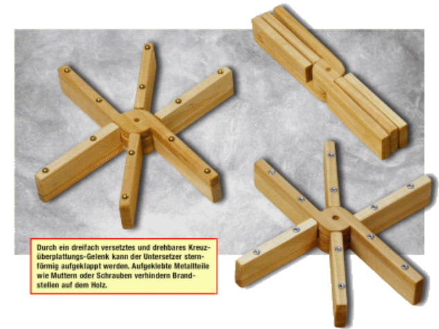
Flügeluntersetzer aus Holz/Metall
